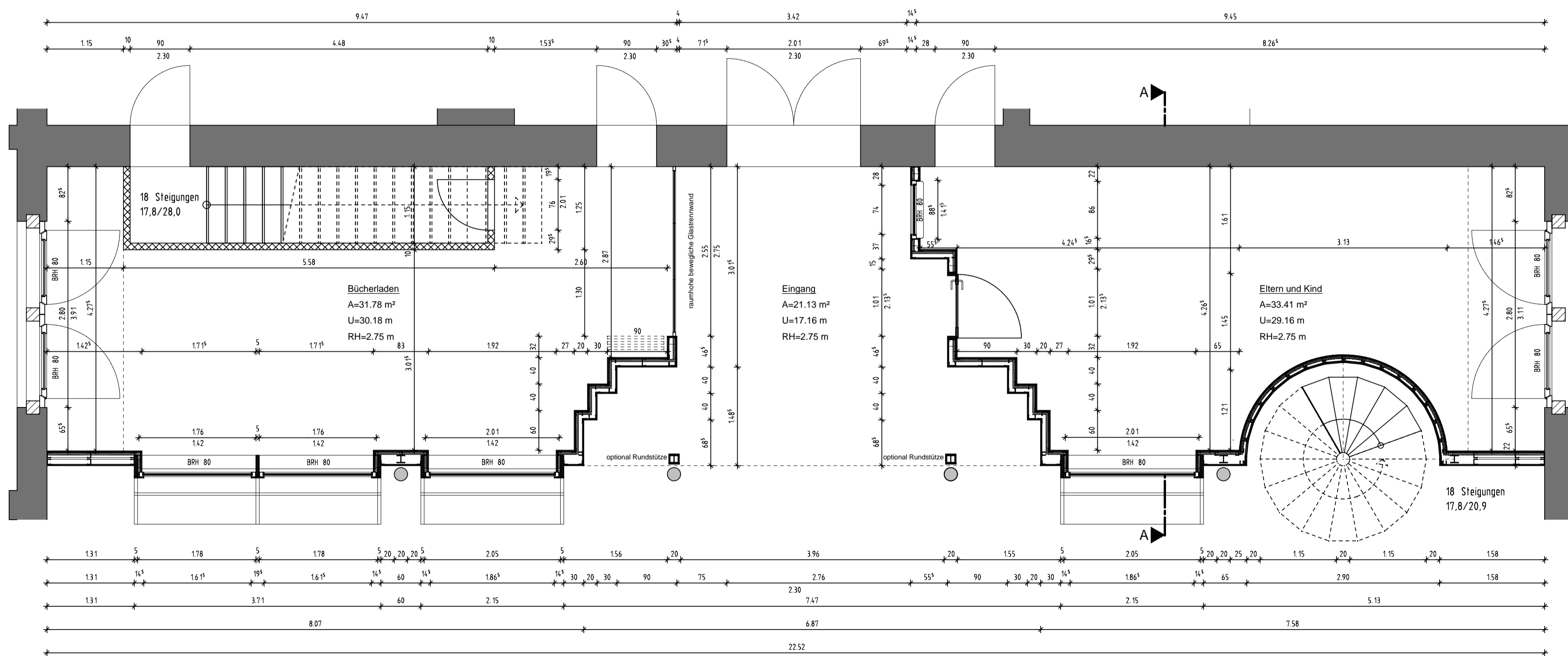
GRUNDRISS
