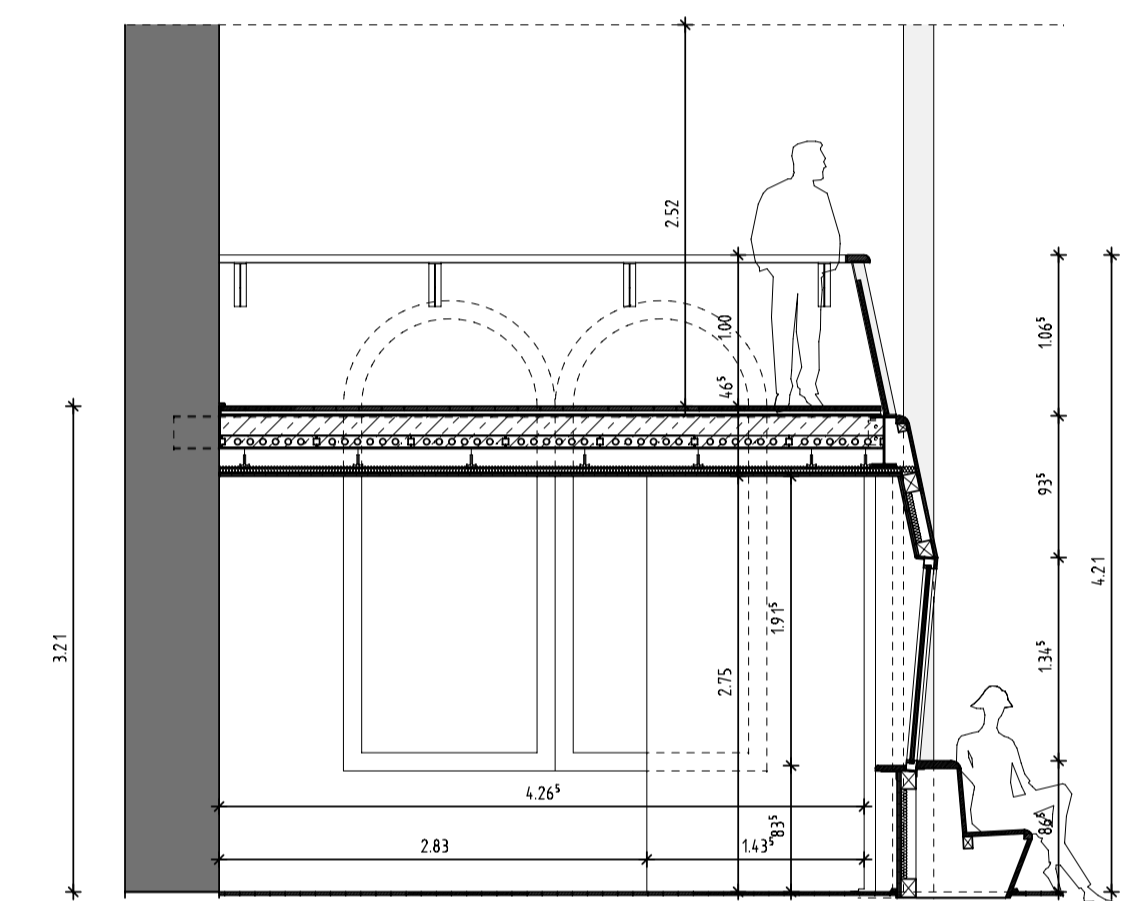
SCHNITT A-A FENSTERFELD
